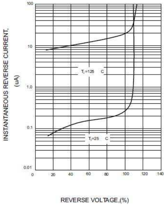
图5. 典型反向特性曲线
