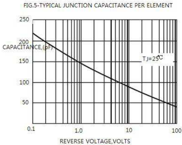
图3. 结电容随反向电压变化曲线
