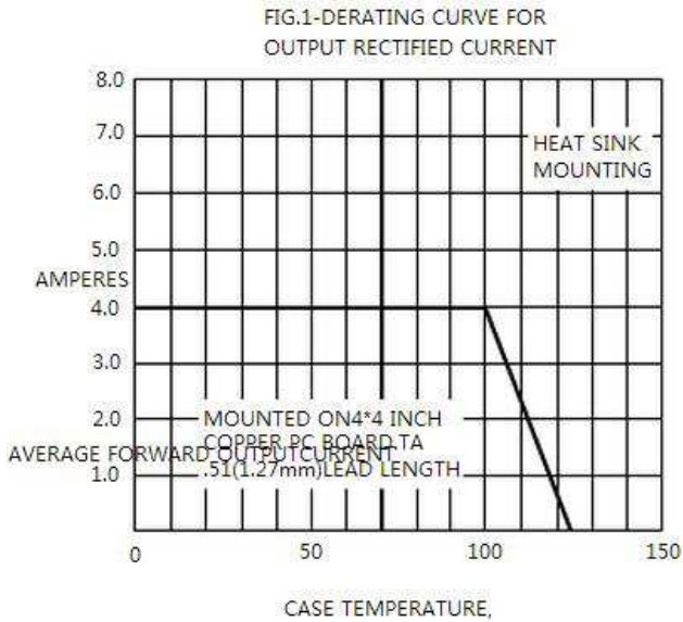
图1. 正向电流随温度变化曲线
