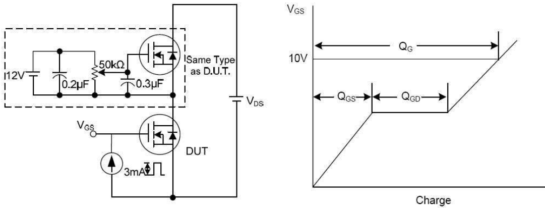
图11. 栅电荷测试
