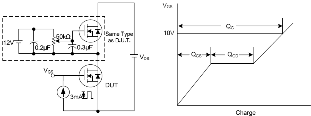
图11. 栅电荷测试
