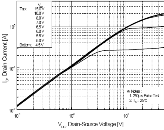
图1. 输出特性曲线 Fig. 1 On-State Characteristics
