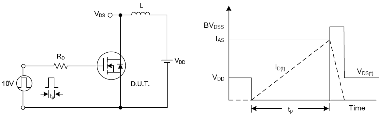
图12. 雪崩能量测试
