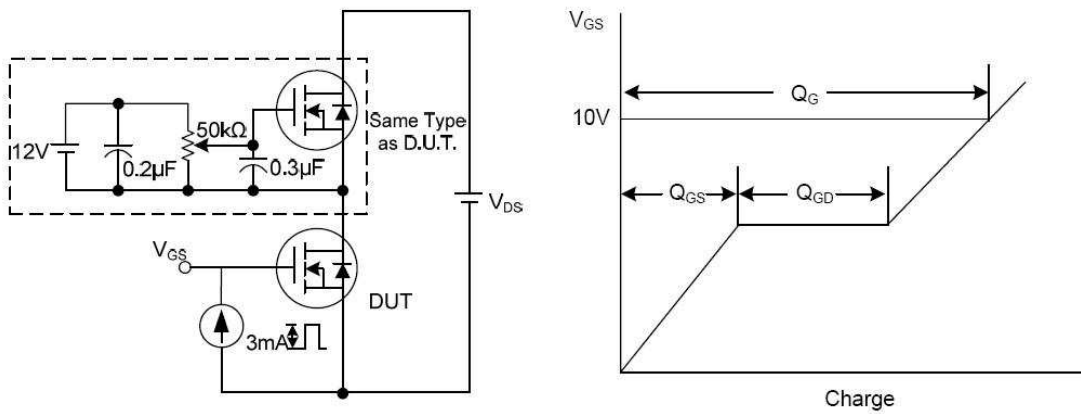
图11. 栅电荷测试
