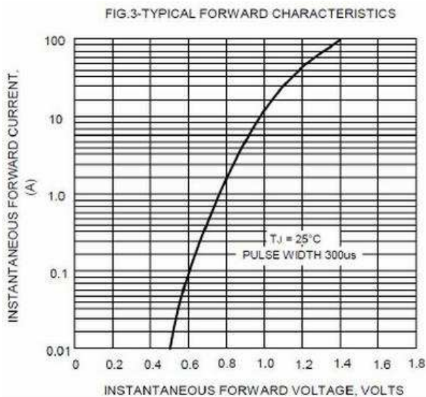
图4. 电性正向特性曲线
