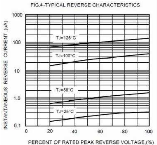
图5. 典型反向特性曲线
